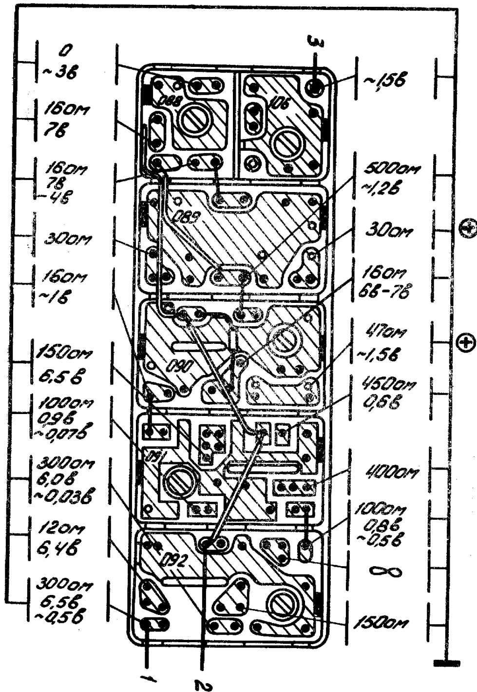
*—«+» прибора на корпусе. Рис. 8. Карта напряжений и сопротивлений. Схема соединений блока А.
