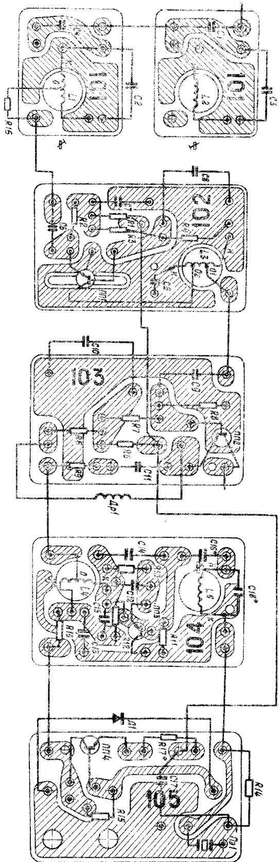
Рис. 20. Схемы соединений плат блока Г.
