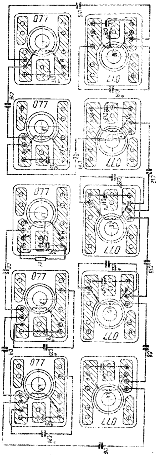
Рис. 22. Схемы соединений плат блока F.
